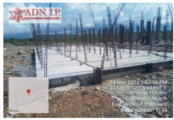
Foto : Penulangan kolom ba Building Dormitorio Soldado.
