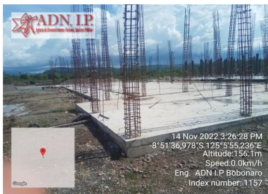
Foto : Penulangan kolom ba Building Dormitorio Soldado
