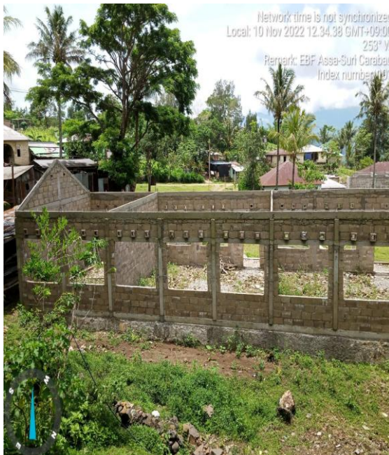
Foto : Servisu monta plat HD ba kuda – kuda
