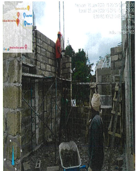
Foto : Servisu pasangan batako.
