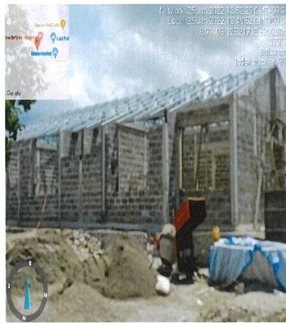
Foto : Pemasangan Kuda – Kuda
