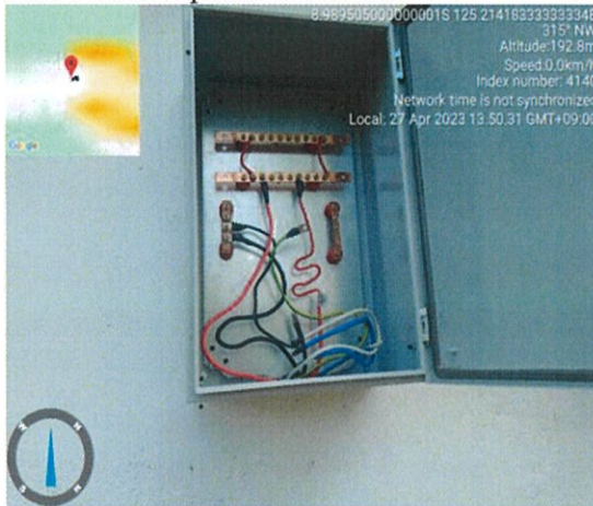
Foto : servisu panel box listrik
