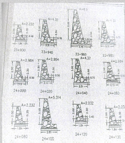
Sketch & Foto Desenho Stone Masonry
