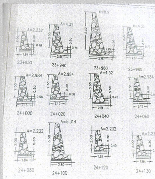
Sketch & Foto Desenho Stone Masonry
